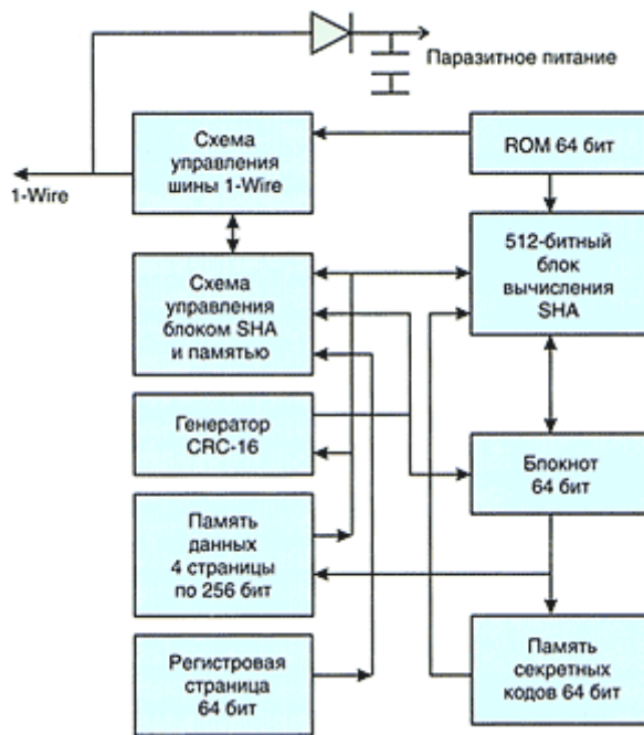
Рис. 1. Структурная схема DS1961S
