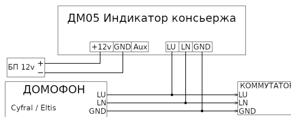
Подключение ДМ-05 к домофону с координатно-матричной адресацией абонентов
