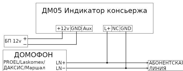
Подключение ДМ-05 к домофону с цифровой адресацией абонентов
